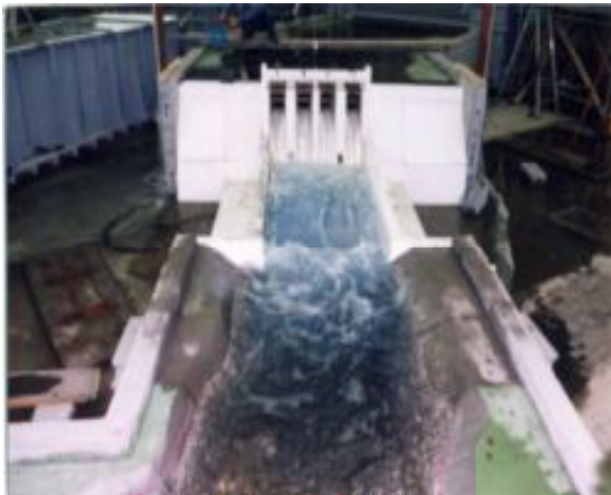
図-1 洪水吐・減勢工の水理実験
