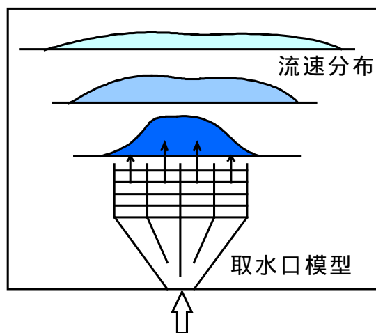
図-3 揚水発電所放水時の放水流均等化実験
